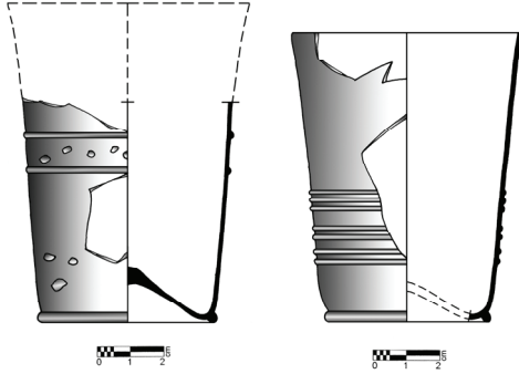
Şek.5-Kadikalesi Kazısı buluntusu iki cam bardağın çizimi (Çizim: Zeynep ORAL ÇAKMAKÇI)
