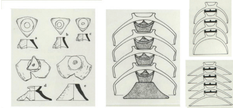
Şek.1-Koniklerin ve üçayakların kullanım biçimleri
