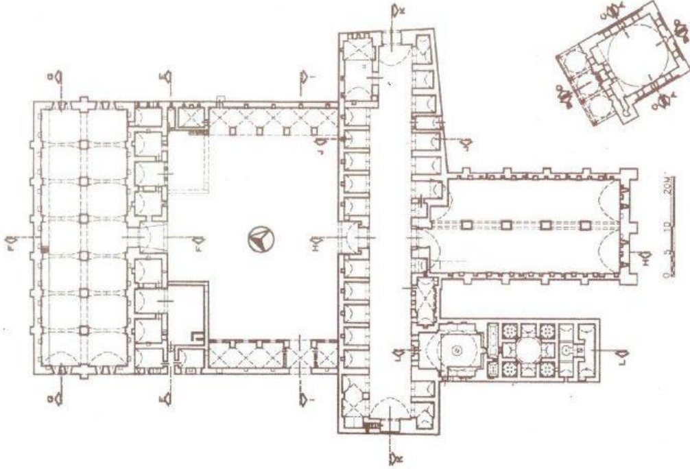
Ek 4: Öküz Mehmed Paşa'nın Ulukışla'da bina eylediği menzil ve planı. Bkz. http://www.trenulukislasi.com/?pnum=29&pt=%C3%96k%C3%BCz+Mehmet+Pa%C5%9Fa+ve+Uluk%C4%B1%C5%9Fla
